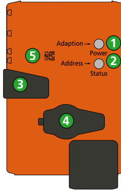
Abb. 1. REACT V BMP-Regler.
