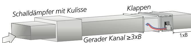
Abb. 9. Anforderungen an gerade Strecken 3 \times B bei Schalldämpfern mit Kulisse. Gilt sowohl für Zu- als auch Abluft.
