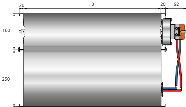
Abb. 7. Abmessungen (mm), REACT V BMP rechteckig.
