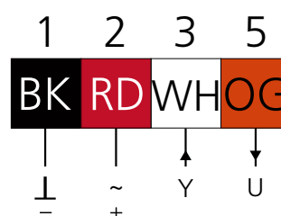
Abb. 2. Anschluss.
