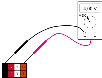
Figur 15. Viser tilkobling av voltmeter for kontroll av erverdi.
