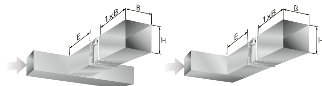
Figur 6. Krav til rett strekning for rektangulære kanaler.
