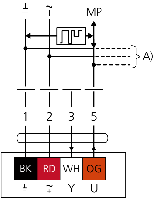
Figur 9. Koblingsskjema MP-Bus.
