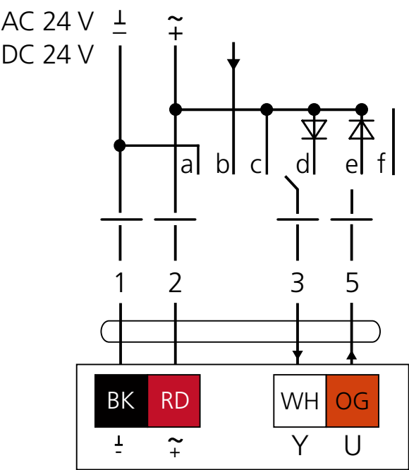
Figur 8. Koblingsskjema.
