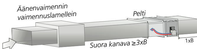
Kuva 7. Suoran kanavan vaatimus 3 \times B äänenvaimentimille. Koskee sekä tulo- että poistoilmaa.
