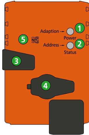
Kuva 10. Belimo-toimilaite.
