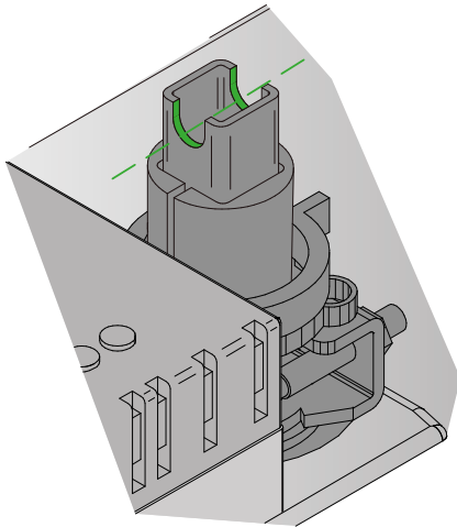
Kuva 17. Ura pellin akselissa osoittaa pellin asennon.
