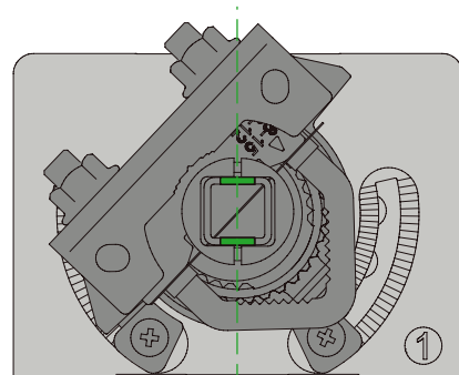
Kuva 18. Pelti auki. Sanka vasemmalle.
