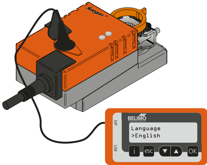
Kuva 14. ZTH EU -käsipäätte toimilaitteen parametrien asettamista ja lukemista varten.
