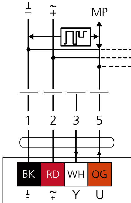
Kuva 9. KytKentäkaavio MP-väylä.
