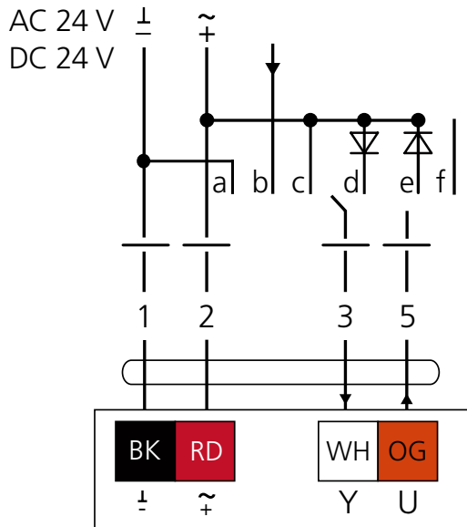
Kuva 8. KytKentäkaavio.
