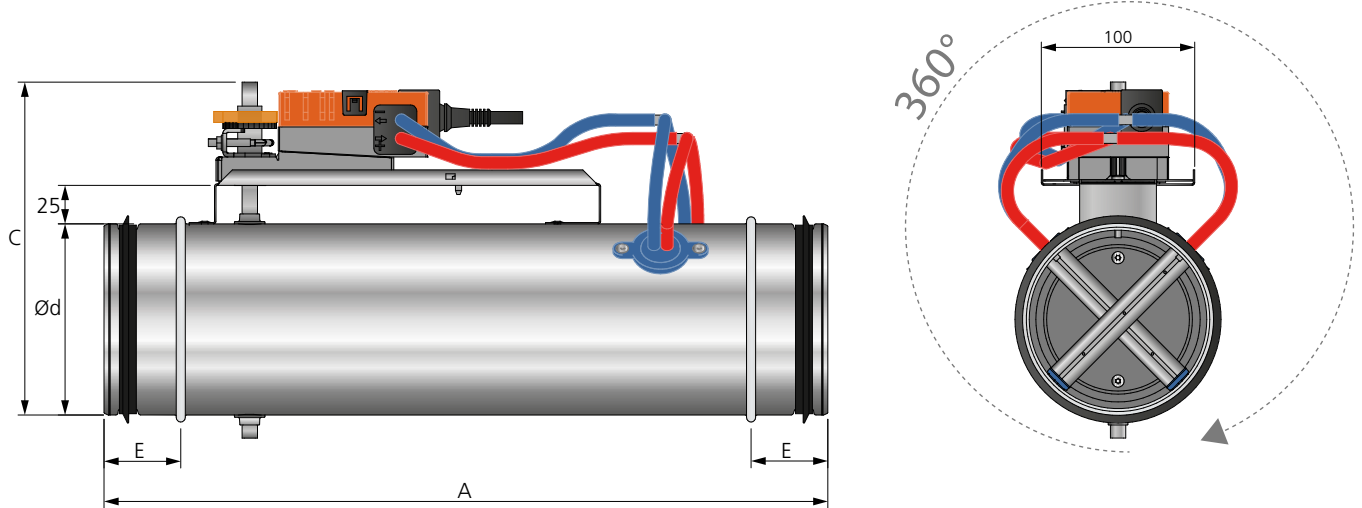
Kuva 1. Mitat (mm), REACT V BMP pyöreä. Pellit voidaan asentaa haluttuunkallistuskulmaan.
