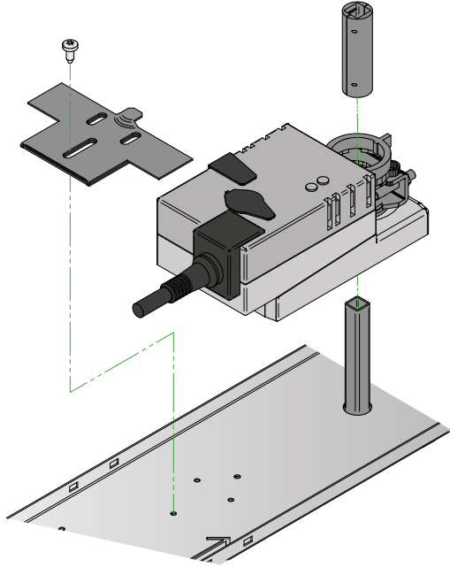
Kuva 16. Peltimoottorin irrotus.
