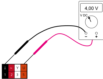
Kuva 15. Näyttää jännitemittarin kytkennän oloarvon tarkistamiseksi.
