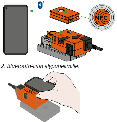
Kuva 13. NFC-liitin älypuhelimille.
