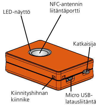
Kuva 11. ZIP-BT-NHC.
