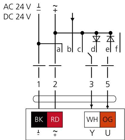
Figur 8. Tilslutningsdiagram.
