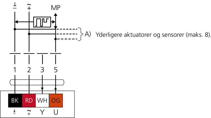
Figur 9. Tilslutningsdiagram MP-Bus.
