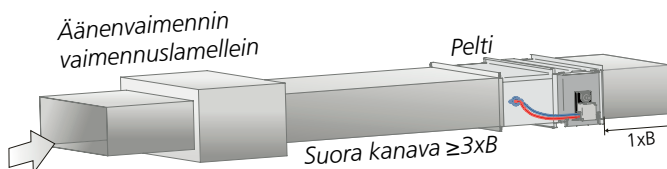
Kuva 9. Suoran kanavan vaatimus 3 \times B äänenvaimentimille. Koskee sekä tulo- että poistoilmaa.
