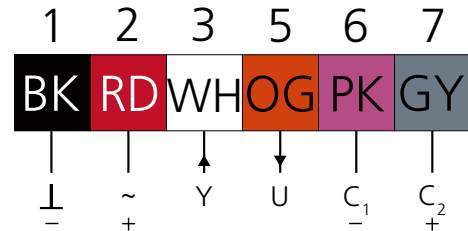
Kuva 2. Kytkenä.
