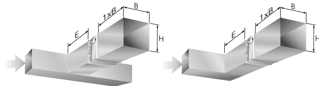
Kuva 8. Vaatimus suorasta kanavasta, suorakaidekanavat.
