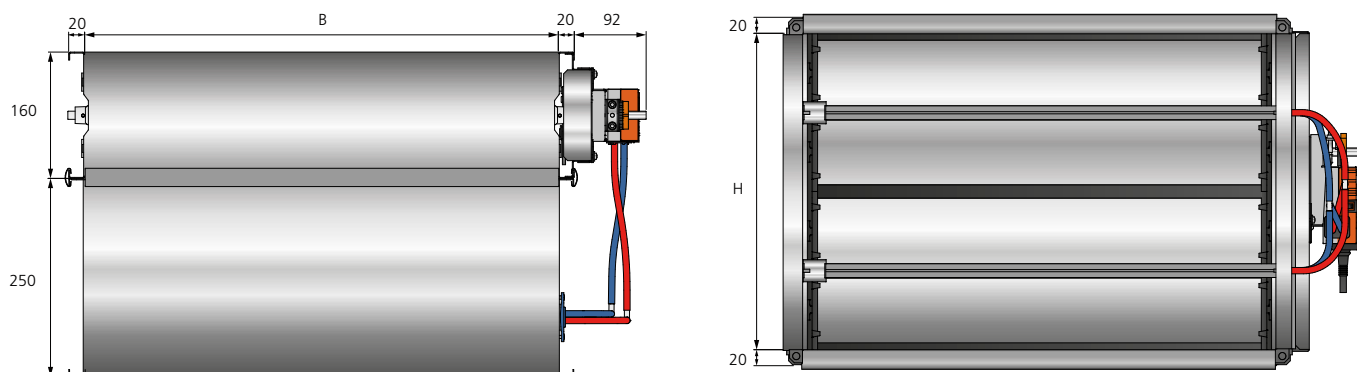
Figur 5. Mål (mm), REACT V BBAC rektangulær.
