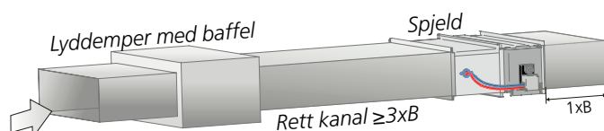
Figur 7. Krav til rettstrekning rektangulær REACT V og lyddemper med baffel. Montering med rettstrekning gjelder både til- og fraluft.
