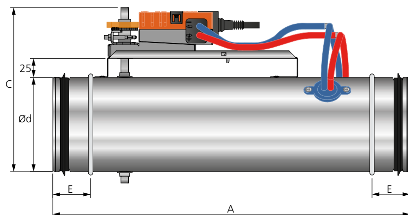
Figur 3. Mål (mm), REACT V BBAC cirkulær. Spjæld kan monteres i valgfri vinkel.
