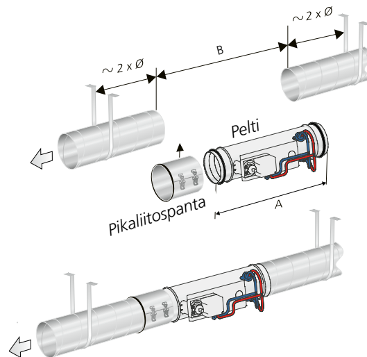
Kuva 4. Asennus kanavistoon. Kanavat pitää kiinnittää rakennuksen runkoon tuotteen molemmiin puoliin.
