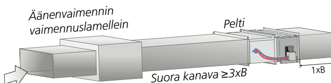
Kuva 7. Suoran kanavan vaatimus 3 \times B äänenvaimentimille. Koskee sekä tulo- että poistoilmaa.
