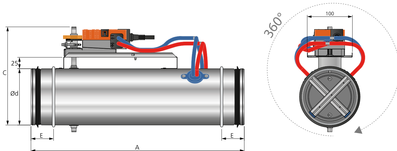
Kuva 1. Mitat (mm), REACT V BBAC pyöreä. Pellit voidaan asentaa haluttuunkallistuskulmaan.
