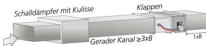
Abb. 7. Anforderungen an gerade Strecken 3 x B bei Schalldämpfern mit Kulissee. Gilt sowohl für Zu- als auch Abluft.
