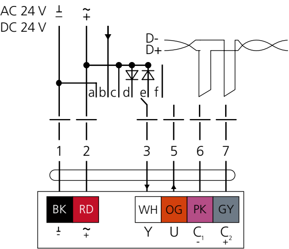
Abb. 8. Schaltplan.
