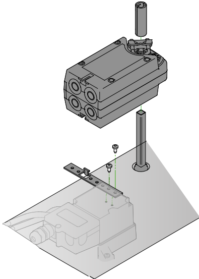
Abb. 8. Demontage des Klappenmotors.
