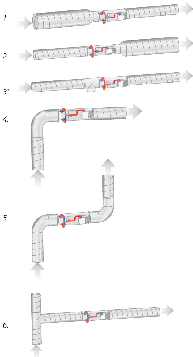
Abb. 2. Anforderung an gerade Strecken, Anzahl Ø vor dem Produkt: Bilder 1–5 erfordern keine gerade Strecke (Bild 3* zeigt ein T-Stück mit Reinigungsdeckel). Bild 6 erfordert eine gerade Strecke vor der Klappe entsprechend 4 x Kanaldurchmesser.
