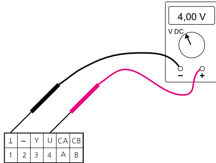
Abb. 7. Zeigt den Anschluss des Voltmeters für die Kontrolle des Istwerts.
