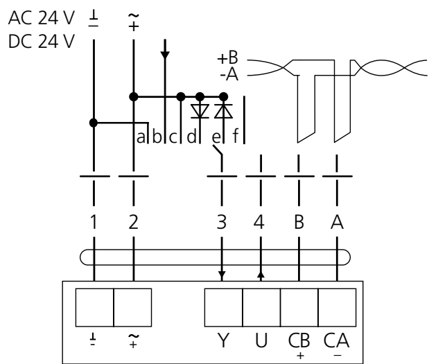
Abb. 5. Schaltplan.
