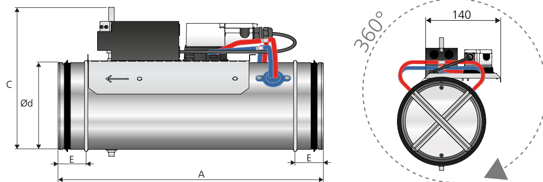
Abb. 1. Abmessungen (mm), REACT V-SR GMB. Die Klappe kann unter einem beliebigen Winkel montiert werden.
