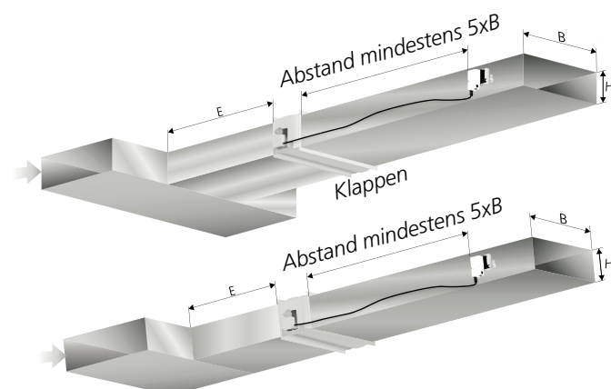
Abb. 8. Anforderung an gerade Strecken und Abstände in rechteckigen Kanälen. E = gerade Strecke B = Breite des Kanals H = Höhe des Kanals
