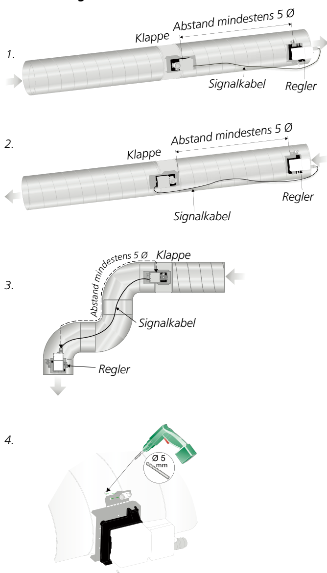
Abb. 5. Anforderung an den Abstand für runde Kanäle, Anzahl Ø vor und hinter dem Produkt:
