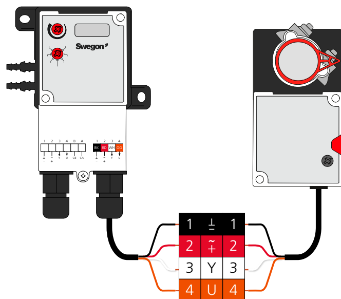
Abb. 4. Anschluss zwischen Stellantrieb und Regler.
