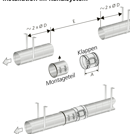
Abb. 6. Installation im Kanalsystem. Die Kanäle müssen in der Gebäudekonstruktion auf jeder Seite des Produkts fixiert werden.
