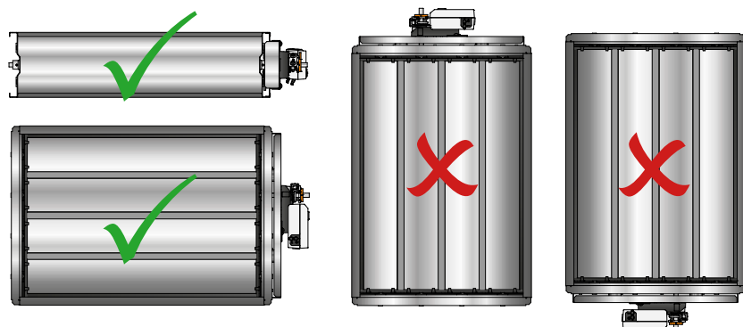
Abb 8. Montage - Für rechteckige Kanäle wird die Klappe stets so montiert, dass der Regler/Stellantrieb sich seitlich in längsrichtung zum Kanal befindet.
