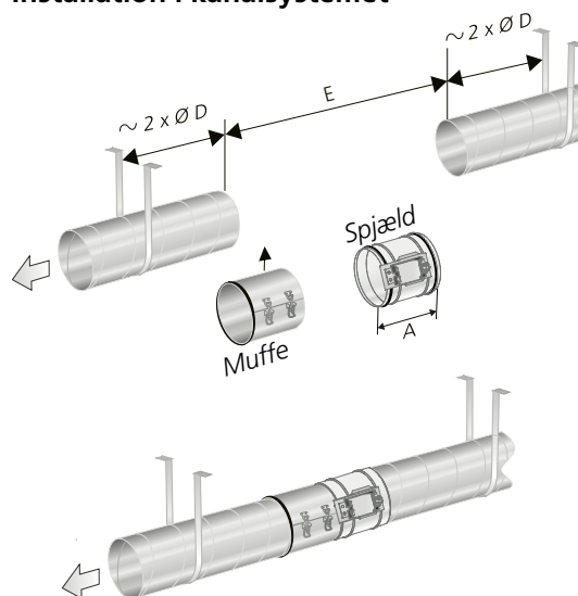
Figur 3. Installation i kanalsystemet. Kanalerne skal fastgøres i bygningens bærende konstruktion på hver side af produktet.
