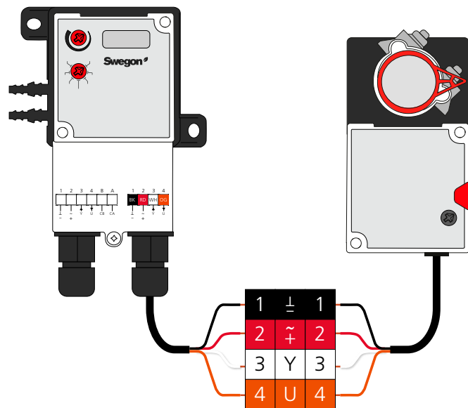
Figur 8. Tilslutning mellem aktuator og regulator.
