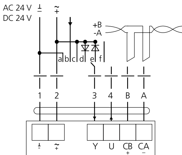
Figur 7. Tilslutning.
