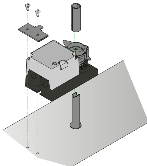
Figur 12. Afmontering af spjældmotor.
