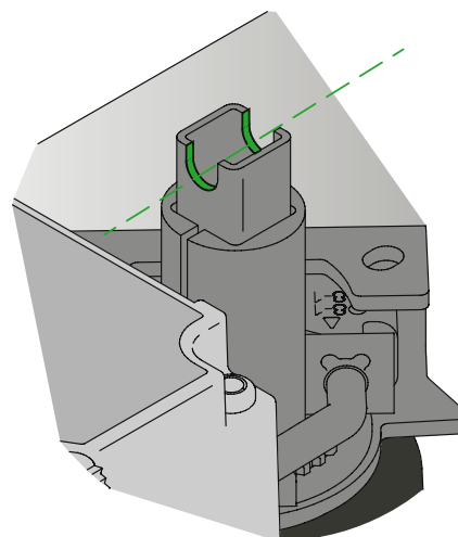
Figur 13. Udclip i spjældaksel angiver spjældets position.
