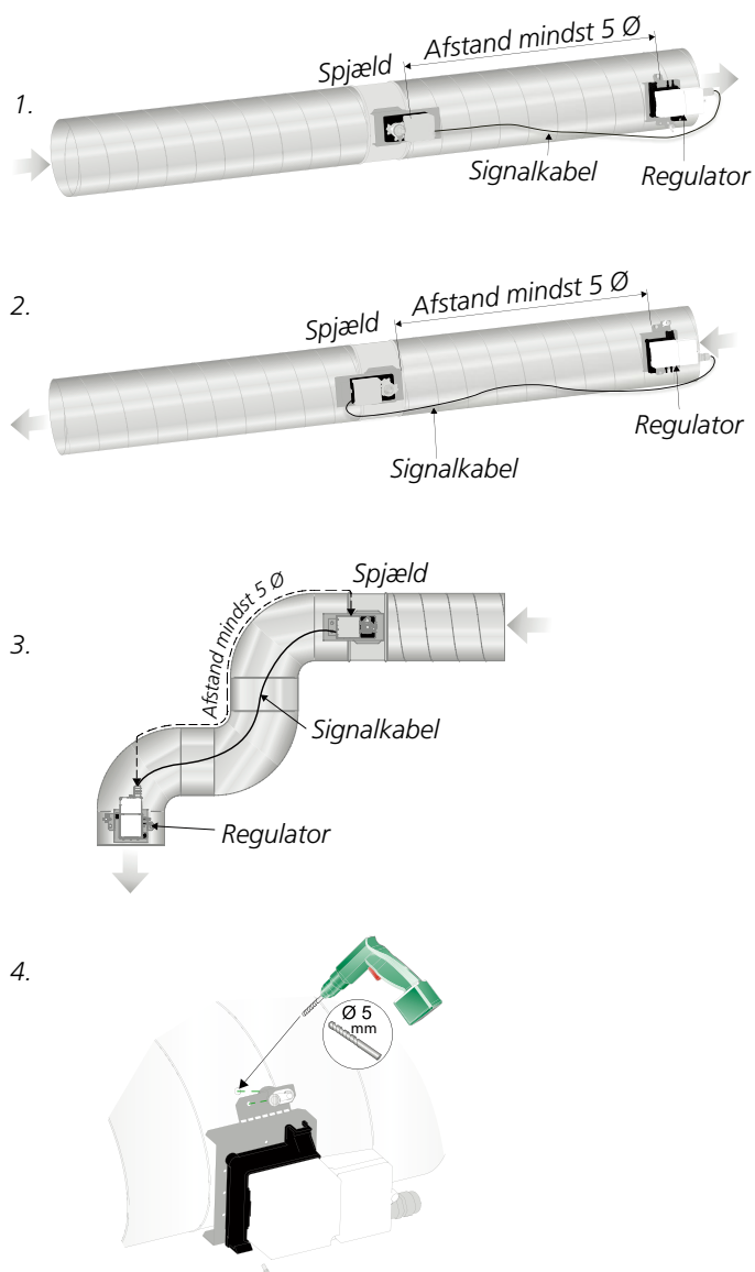
Figur 2. Afstandskrav i cirkulære kanaler, antal Ø før og efter produkt:
