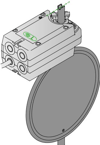
Figur 11. Spjäll öppet med bygel mot vänster (NO).
