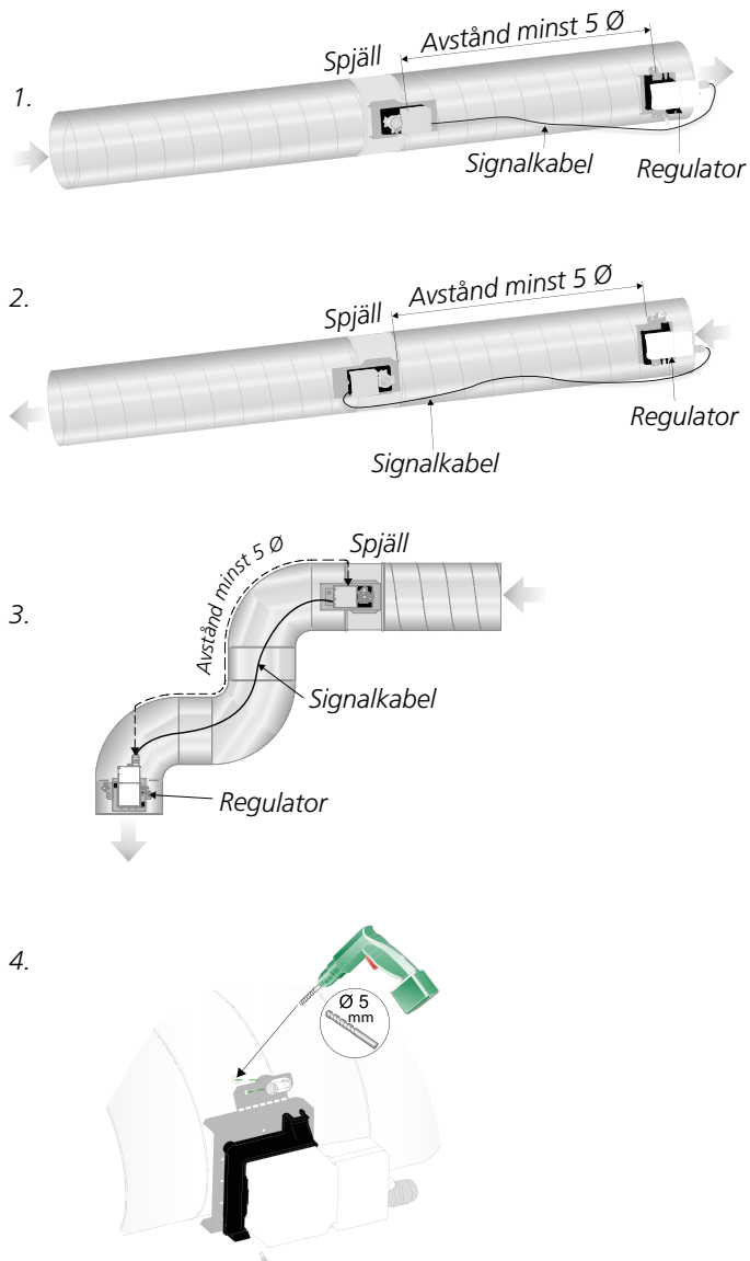
Figur 2. Krav på avstånd, antal Ø före och efter produkt:
