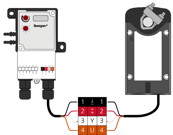
Figur 5. Inkoppling mellan ställdon och regulator.
