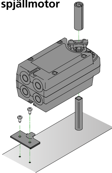
Figur 9. Demontering av spjällmotor.
