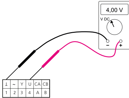
Figur 8. Visar inkoppling av voltmeter för kontroll av ärvärde.
