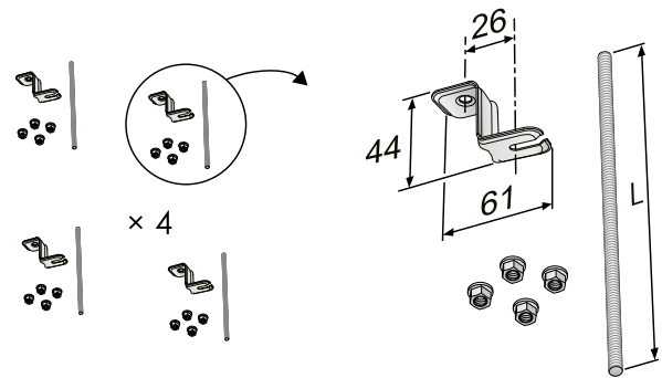
Abb. 17. Montageteil SYST MS M8-1, Deckenbefestigung und Gewindestange
