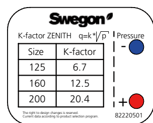
Abb. 24. Etikett mit K-Faktor-Werten.
