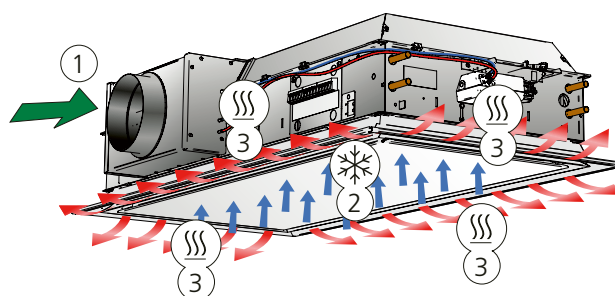
Abb. 3. Ausführung B: Heiz- und Zuluftfunktion
