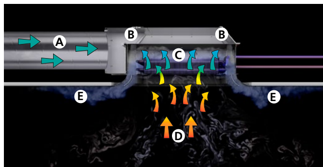
Abb. 4. Das Induktionsprinzip in REACT Parasol Zenith
