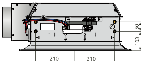
Abb. 22. Abmessungen, Wasseranschluss Länge 600, 1200, 1800
