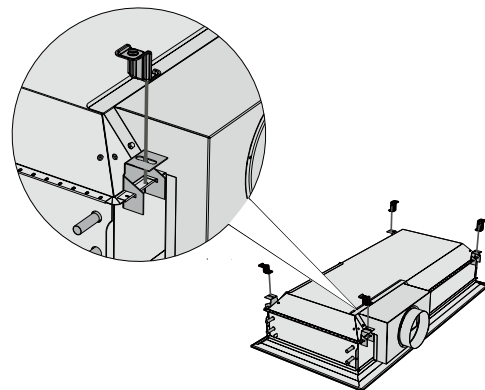
Abb. 18. Aufhängung an vier Befestigungen mit SYST MS M8
