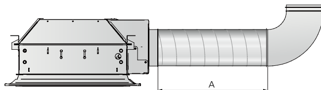
Abb. 25. Maßskizze, Anschluss an der langen Seite mit Bogenj
