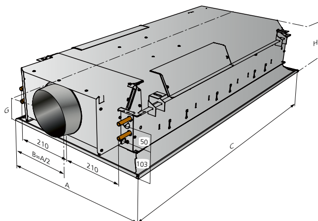
Abb. 27. Maßskizze – Anschluss an einer kurzen Seite (im Beispiel wird die Länge 1200 mit Luftanschluss an Seite 1 gezeigt).
