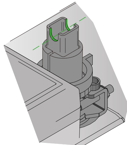
Figur 12. Udklip i spjældaksel angiver spjældets position.
