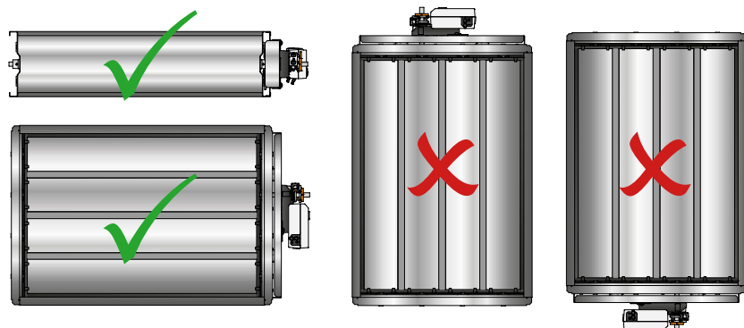
Figur 5. Montering - For rektangulære kanaler monteres spjældet altid således at regulatoren/aktuatoren er placeret langs med siden af kanalen.
