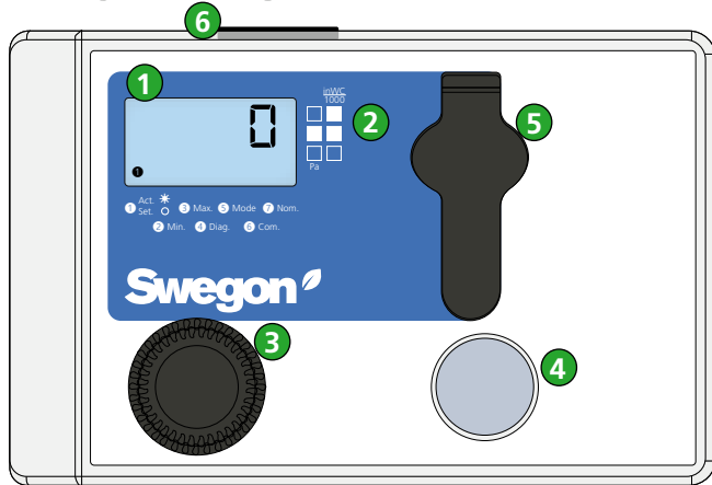
Figur 9. Gruner-aktuator.
