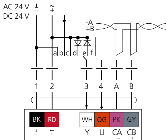
Figur 7. Tilslutningsdiagram.
