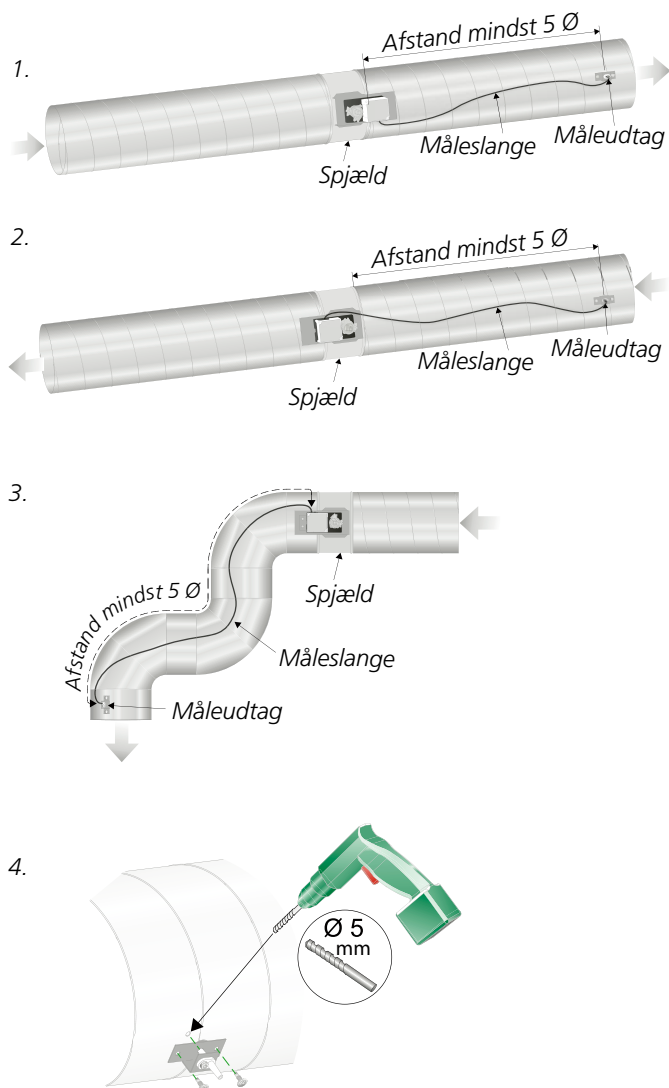
Figur 2. Krav til afstand i cirkulære kanaler, antal Ø før og efter produkt:
