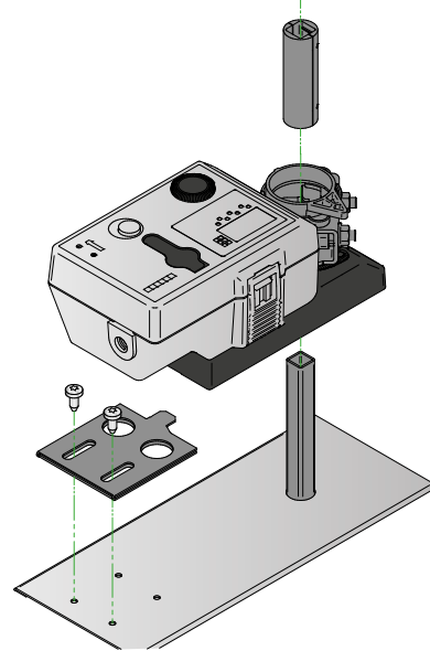
Figur 11. Afmontering af spjældmotor.
