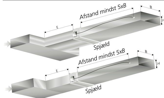
Figur 6. Krav til lige strækninger og afstand i rektangulære kanaler.
