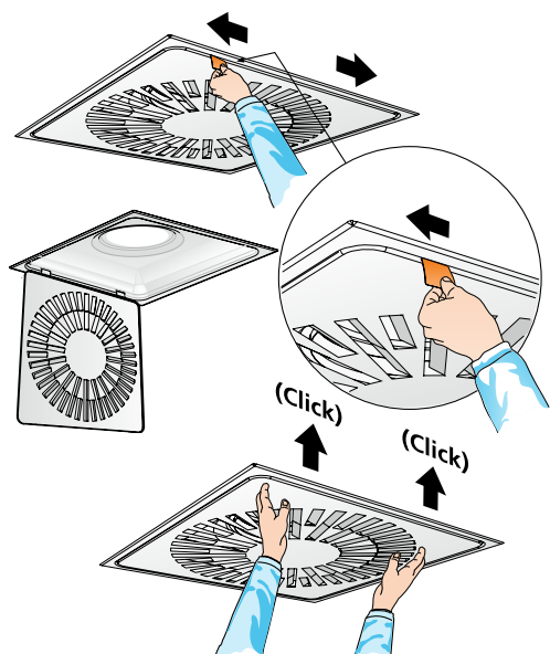
Abbildung 2. Quick Access, demontage der Front.
