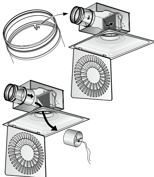
Abbildung 4. Demontage der Klappe
