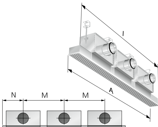
Abbildung 5. SRY mit drei Anschlusskästen.
