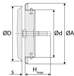
Abb. 6. TRAC, Abmessungen.
