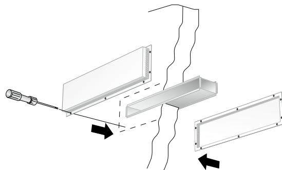
Abb. 1. ROT, Montage
