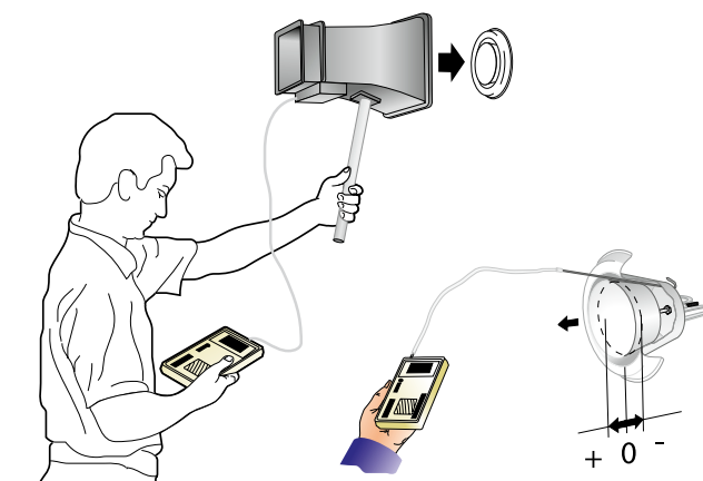
Abb. 3. Einregulierung.
