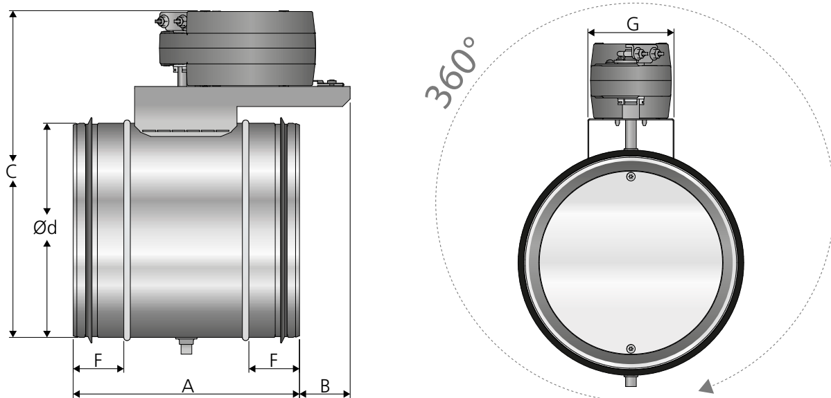
Abb. 5. Abmessungen (mm), REACT PX-SR GMB. Die Klappe kann unter einem beliebigen Winkel montiert werden.
