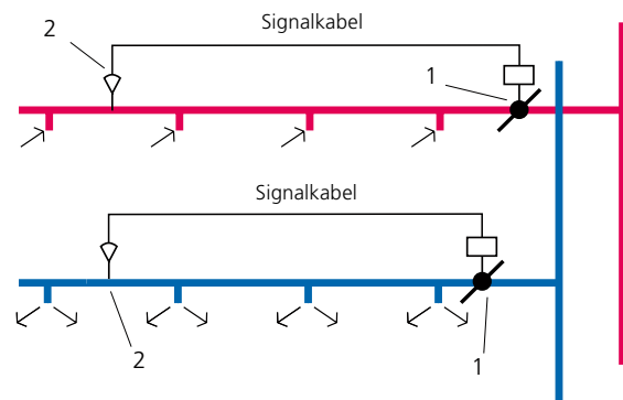
Abb. 2. Druckregelung.
