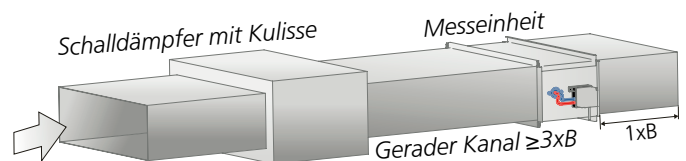
Abb. 9. Anforderungen an gerade Strecken 3 \times B bei Schalldämpfern mit Kulissen. Gilt sowohl für Zu- als auch Abluft.
