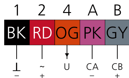
Abb. 2. Anschluss.
