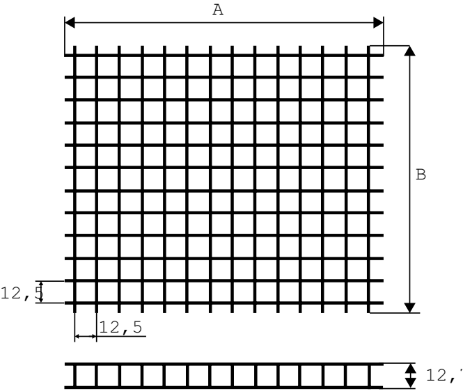
Abb. 3. Abmessungen RASTER.
