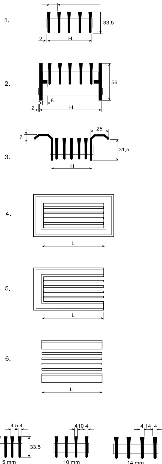
Abbildung 3. Maße.
