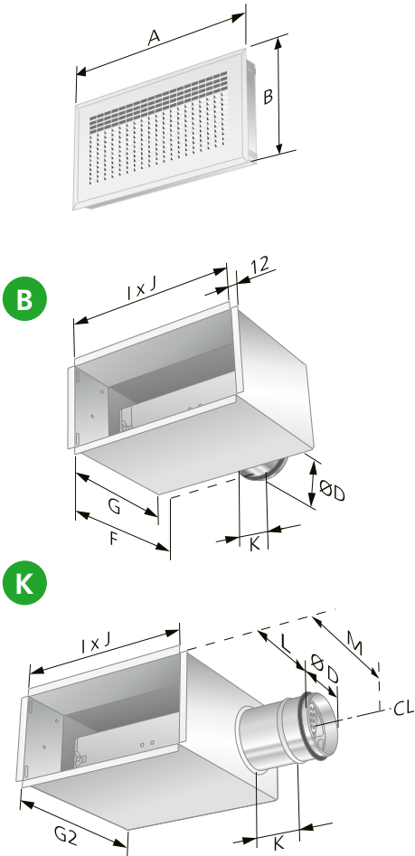
Abb. 4. Abmessungen, LOCKZONE Wall und Anschlusskasten ALV. B = Anschluss an der Rückseite. K = Anschluss an der Kurzseite. CL = Mittellinie.
