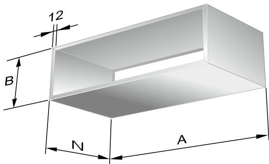
Abb. 3. Abdeckblech ALVT 1.
