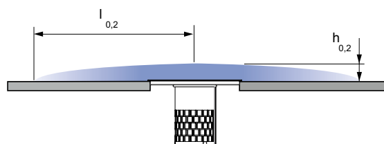
Abbildung 4. Isovel, Strahlhüllgrenze.
