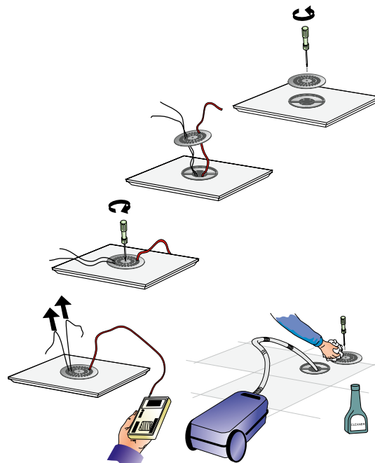
Abbildung 2. Montage. Wartung.
