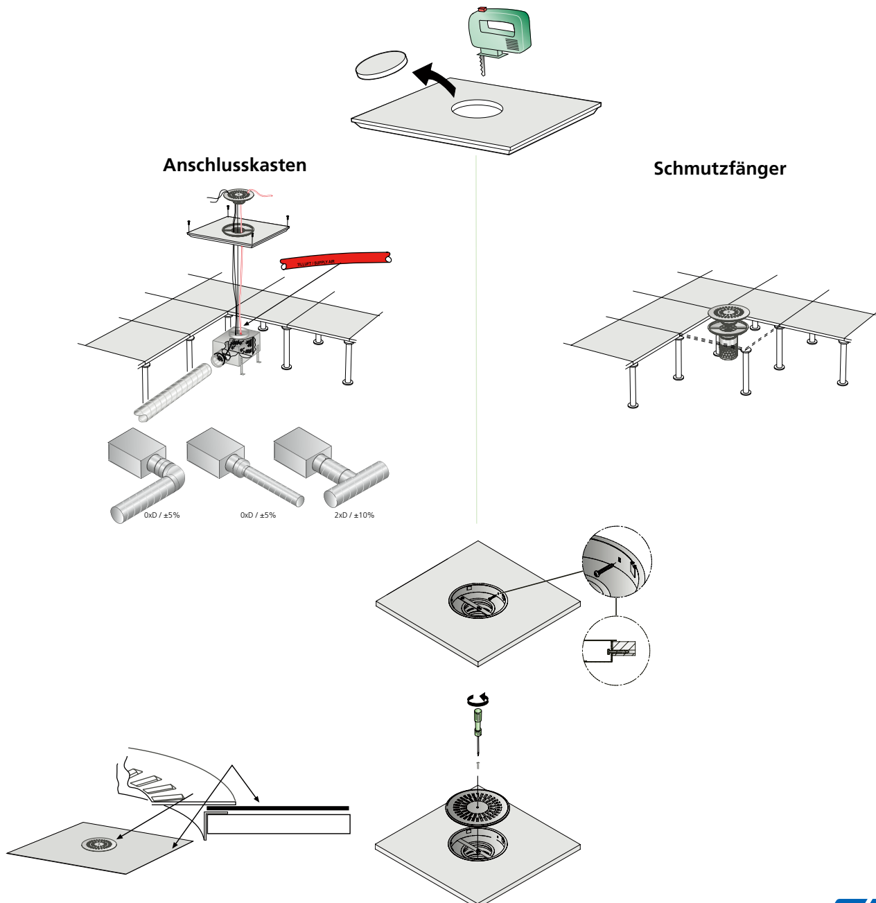
Abbildung 1. Montage.
