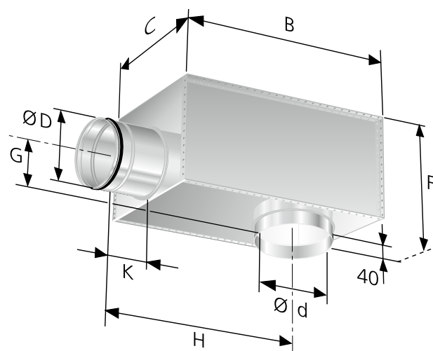
Abbildung 5. Anschlusskasten, ALS.
