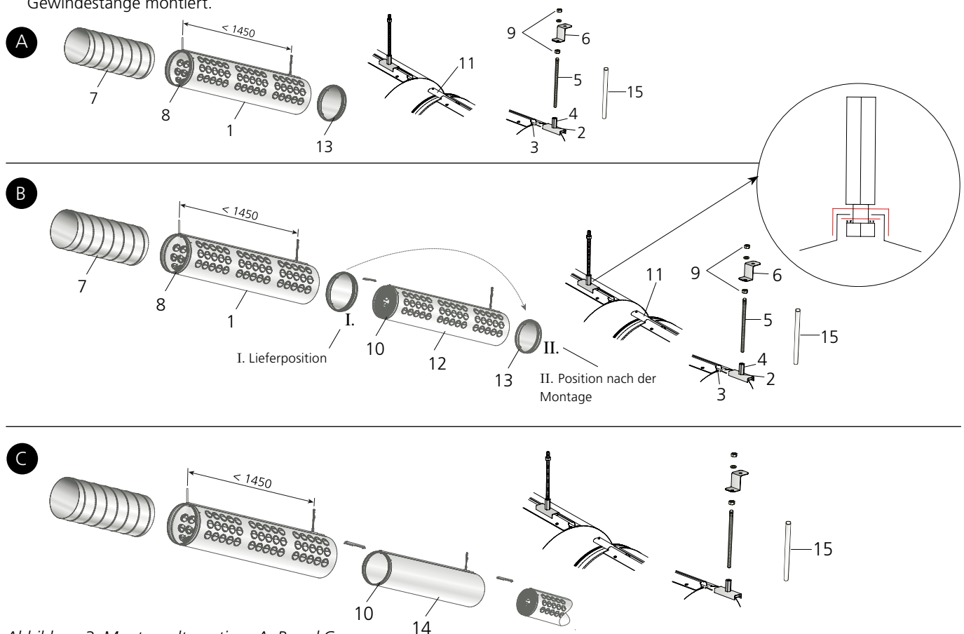
Abbildung 3. Montagealternativen A, B und C.
