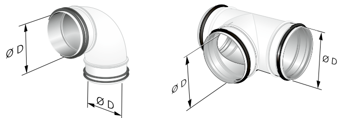
Abbildung 12. IBIS B und IBIS T.
