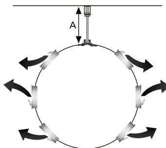
Abbildung 6. Zweiseitige Ausblasrichtung mit langer Wurfweite. Die obersten Düsenreihen müssen auf beiden Seiten der Montageschiene nach unten ausgerichtet sein.
