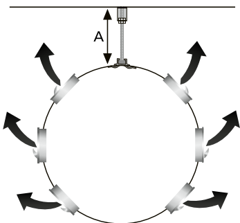
Abbildung 5. Zweiseitige Ausblasrichtung mit kurzer Wurfweite. Alle Düsen werden nach oben zur Montageschiene ausgerichtet.
