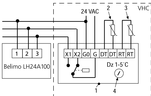
Abbildung 4. Das Anschlussdiagramm zeigt den Anschluss mit Belimo Klappenstellmotor zum VHC. BEACHTEN! Funktioniert nur mit 24 V AC Netzteil.
