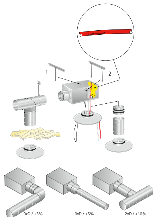
Abbildung 1. Montage Einregulierung.
