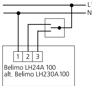
Abbildung 4. Anschlussdiagramm für FALCON C mit Motorsteuerung mit 3-Punktregelung Umschalter nicht im Lieferumfang enthalten.
