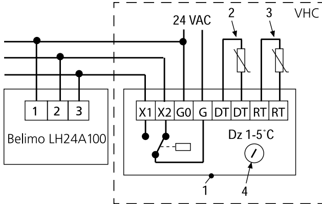
Abbildung 5. Das Anschlussdiagramm zeigt den Anschluss mit Belimo Klappenstellmotor zum VHC. BEACHTEN! Funktioniert nur mit 24 V AC Netzteil.
