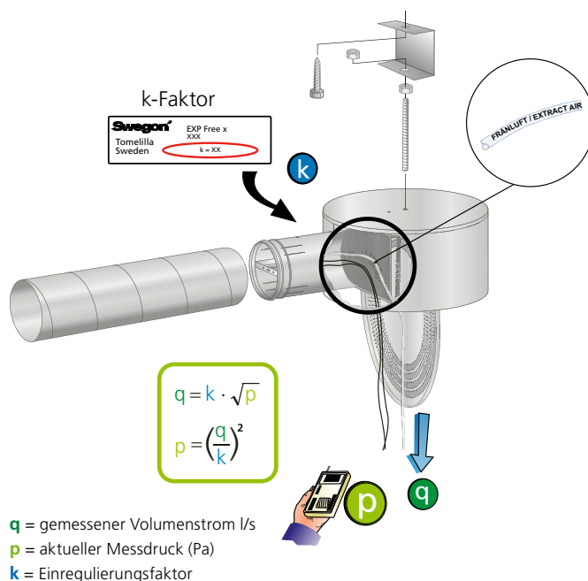
Abb. 1. Montage. Einregulierung. Instandhaltung.
