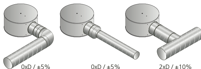
Abb. 2. Anströmlänge.
