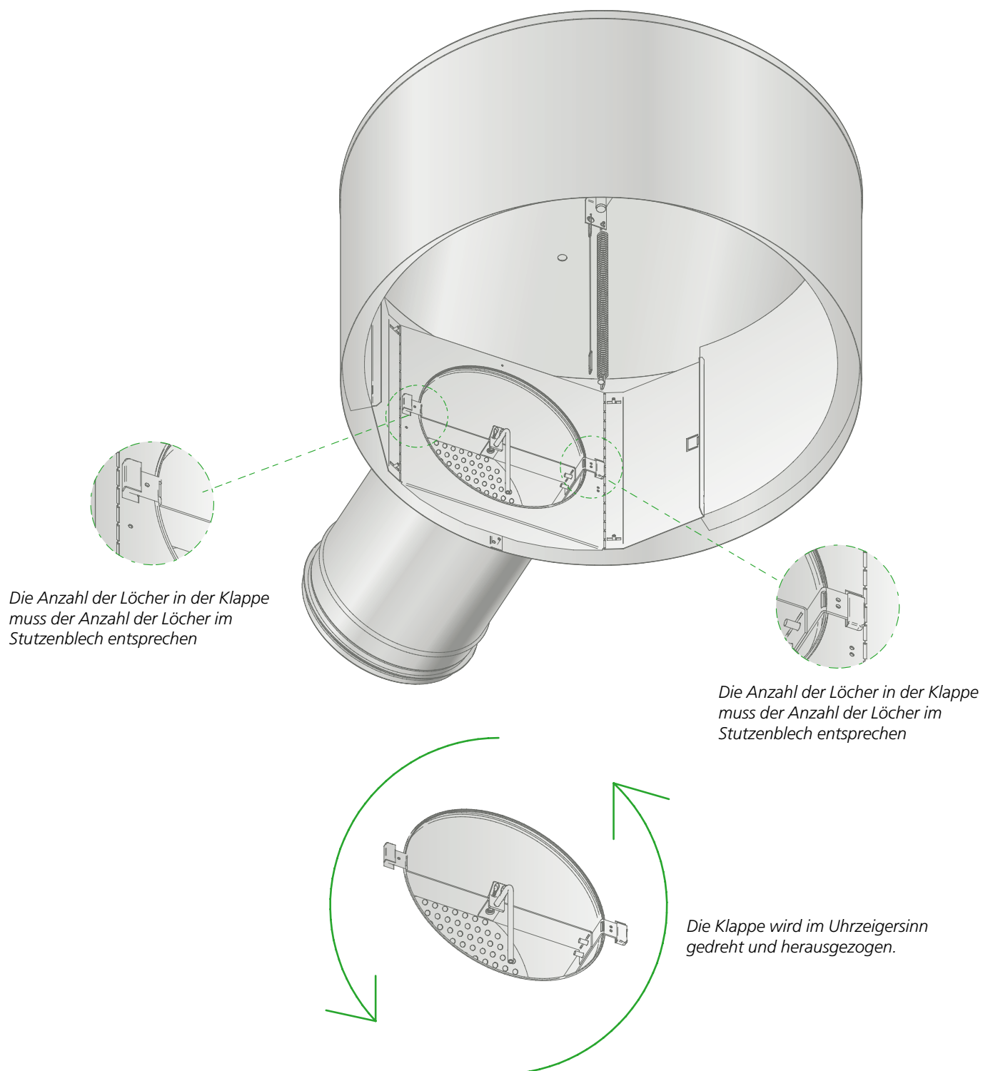
Abbildung 6. Montage und Demontage von Klappen.
