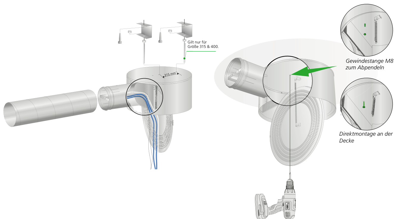
Abbildung 3b. Alternative Montage in vorgestanztem Loch mit Ø10 mm.
