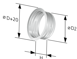
Abb. 6. Befestigungsrahmen EXCT 3. Konischer Befestigungsrahmen für den Anschluss direkt an ein mit einem Nippel versehenes Kanalteile, z. B. einen Kanalbogen.
