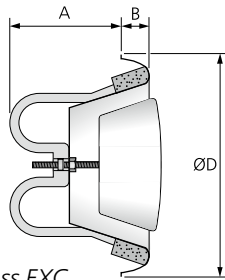
Abb. 4. Abluftauslass EXC.
