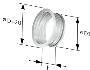
Abb. 5. Befestigungsrahmen EXCT 2.
