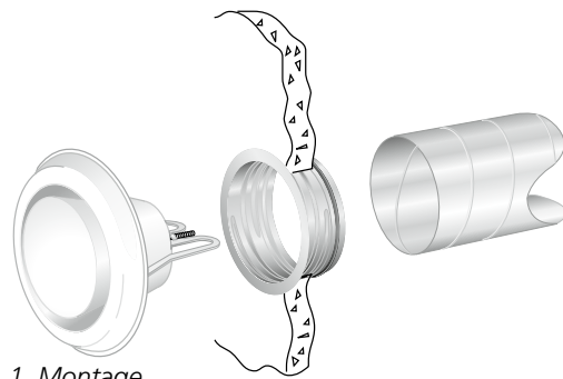
Abb. 1. Montage
