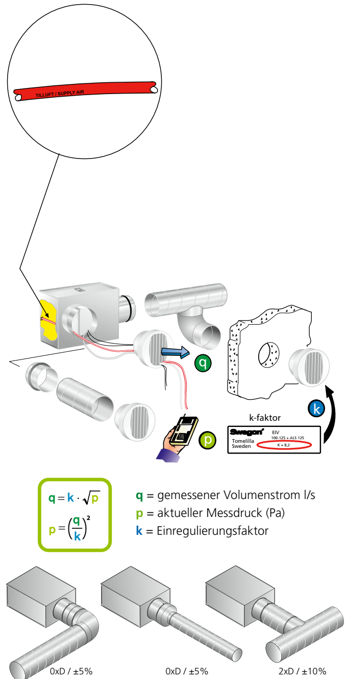
Abbildung 1. Montage Einregulierung.
