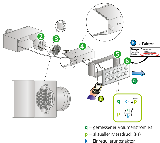
Abb. 1. Montage, Einregulierung.
