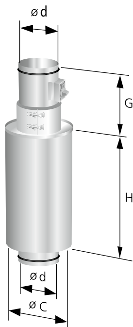
Abbildung 4. Regulierungseinheit REG.
