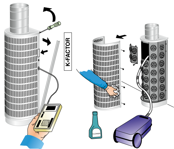
Abbildung 2. Einregulierung. Wartung.
