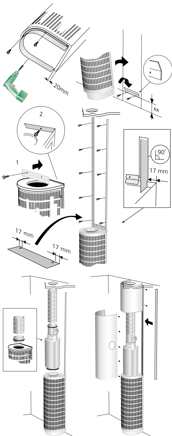
Abbildung 2. Einregulierung. Wartung.
