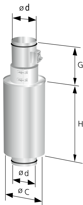
Abbildung 4. Reguliereinheit REG.
