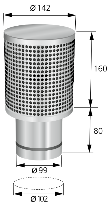
Abbildung 4. DCC. Maßeinheit = mm. Gewicht: 1,2 kg. Ausschnittmaße = Ø102 mm.
