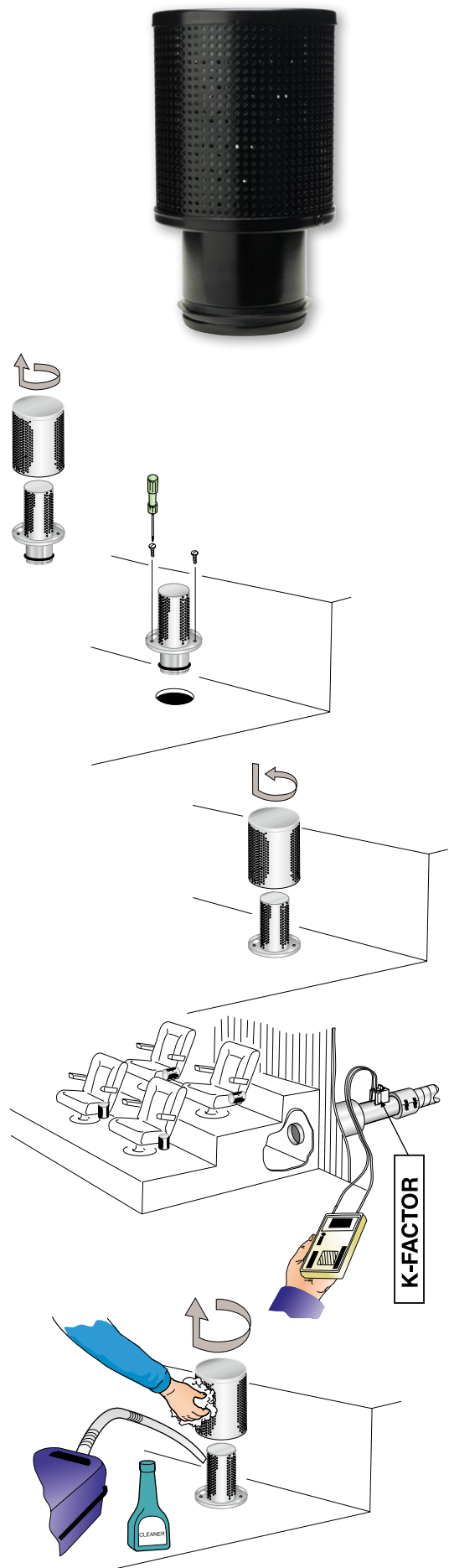
Abbildung 2. Montage. Einregulierung. Wartung.
