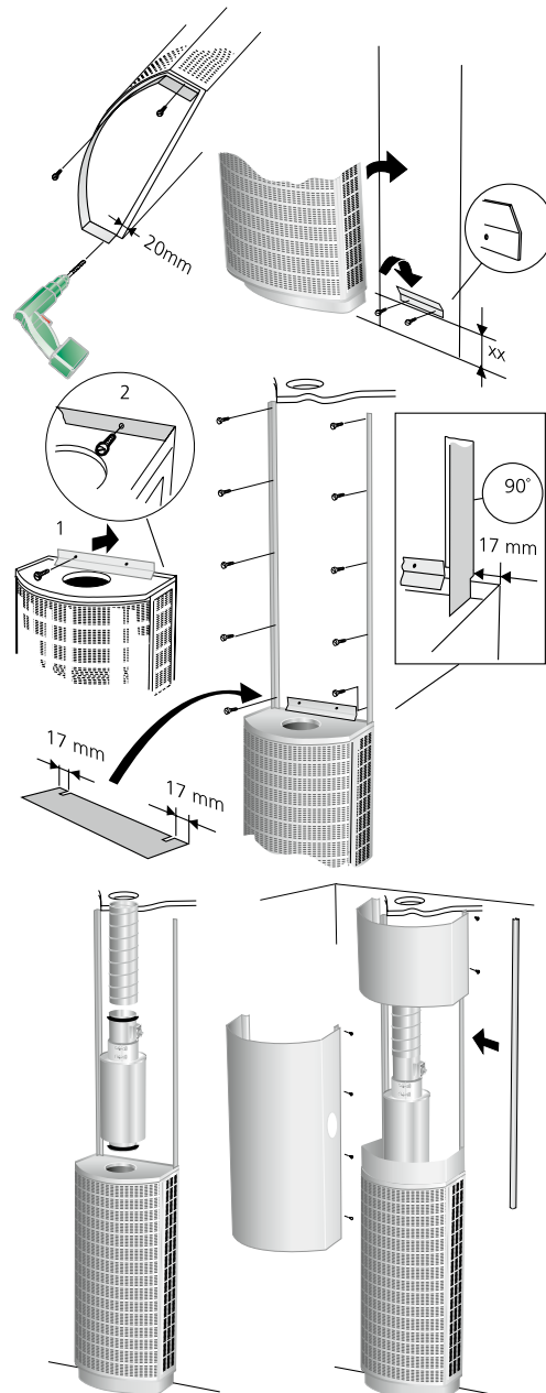
Abbildung 1. Montage.
