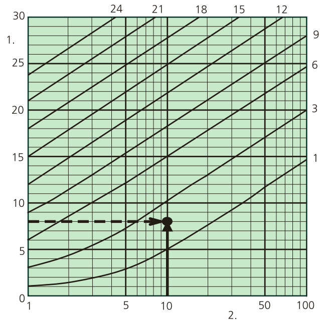
Diagramm 3. Reduktion des Schalldämm-Maßes der Wand, wenn in diese eine Schallkulisserfläche für Überströmung eingesetzt wird.
