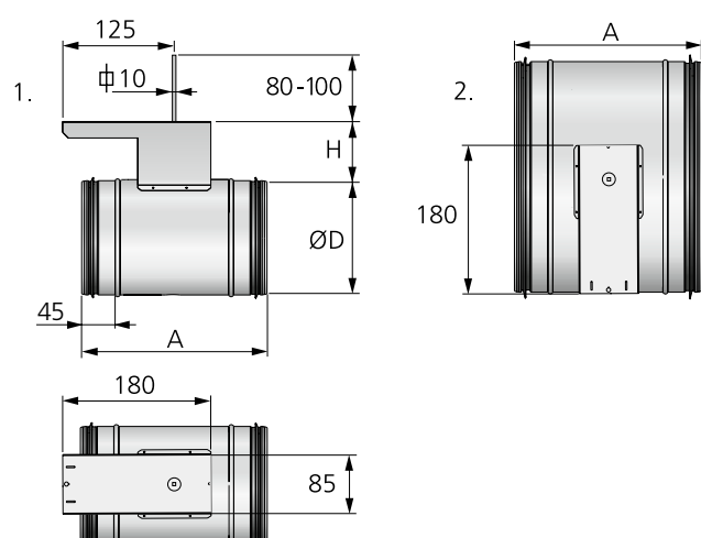
Abbildung 2. Maße (mm), CRT.
