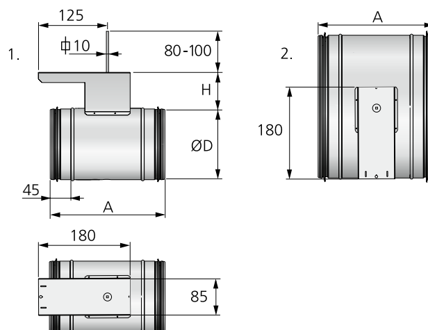
Abbildung 12. Maße (mm), CRP. 1. CRP-(100-400)-4 2. CRP-(500-630)-4
