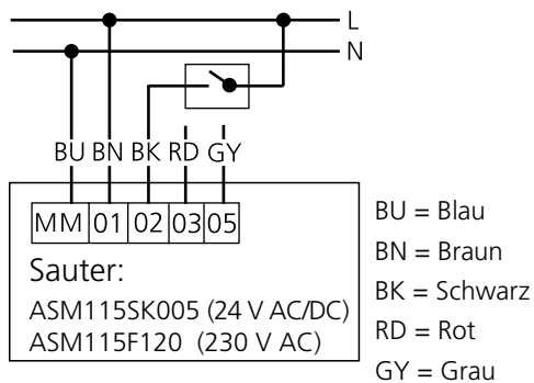
Abbildung 4. Schaltplan Sauter, 2-punktregelung.
