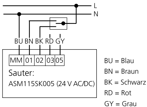
Abbildung 5. Schaltplan Sauter, 3-punktregelung.
