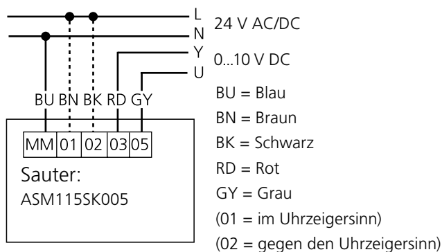
Abbildung 6. Schaltplan Sauter, 0-10 V stufenlos / modulierende Regelung.
