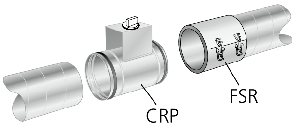
Abbildung 1. Montage.
