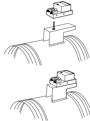
Abbildung 3. Motor montage, größe 100-400.
