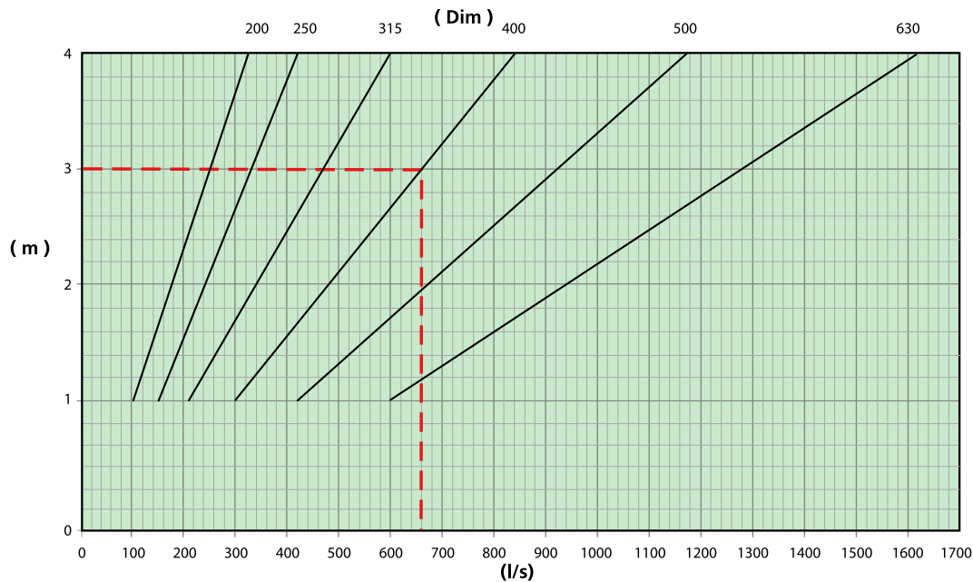
Diagramm 1. Eindringtiefe (m) bei +5 K übertemperatur.
