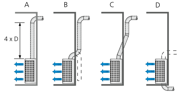
Abbildung 4. Beispiel für die Beeinflussung der Geräuscherzeugung seitens verschiedener Auslassanschlüsse.
