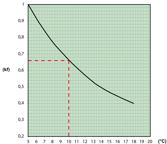
Diagramm 2. Korrekturfaktor andere Übertemperaturen (kf)
