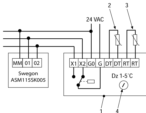
Abbildung 3. Der Schaltplan zeigt den Anschluss zum Zuluftauslass mit Sauters Klappenmotor, der auf einem BOC montiert ist.
