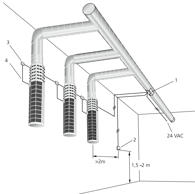
Abbildung 2. BOC mit VHC.
