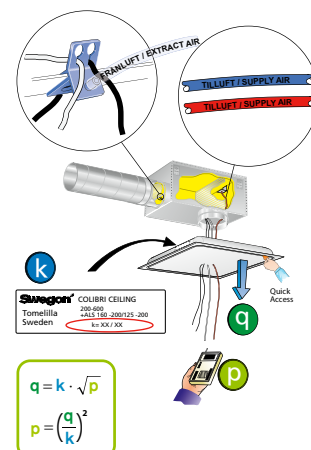
Abbildung 2. Messschläuche für Einregulierung
