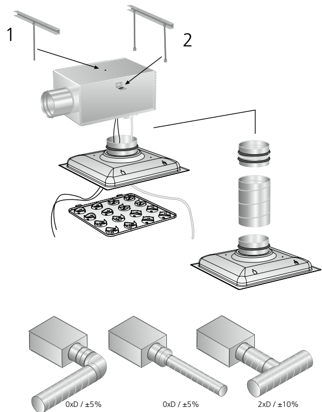
Abbildung 1. Montage.
