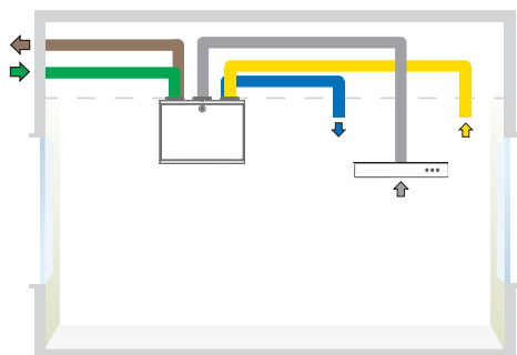
CASA W4 xs L, kanaltilkoblinger og kjøkkenhette koblet til ventilasjons- aggregatets kjøkkenkanaltilkobling.
