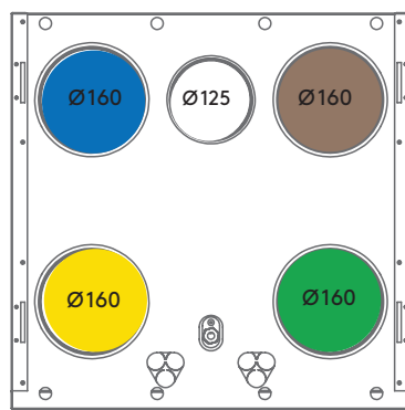
CASA W4 Smart xs R, (høyreutførelse)
