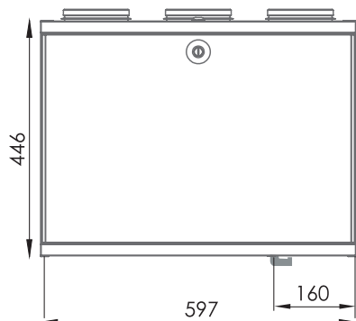
R -modell forfra
