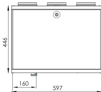
L-modell von vorne
