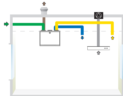
CASA W4 xs L, Kanalanschlüsse und Dunstabzugshaube angeschlossen an einem externen Deckenventilator.
