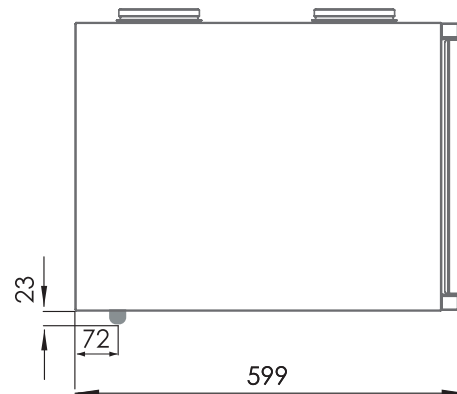
L/R-modell von der seite
