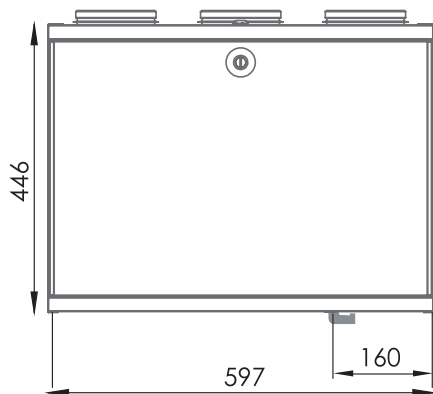
R-modell von vorne
