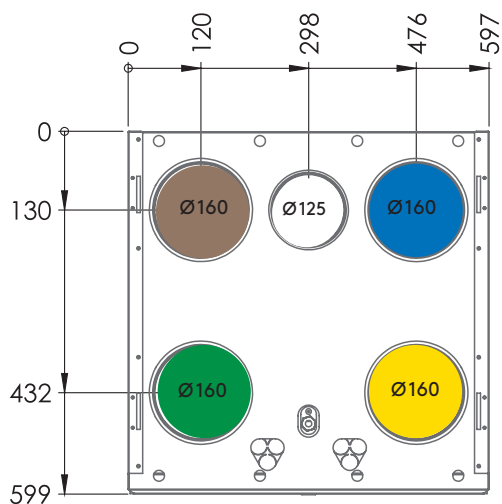
CASA W4 Smart xs L, Linksausführung
