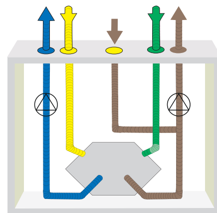
CASA W4 Smart xs L, Rechtsausführung
