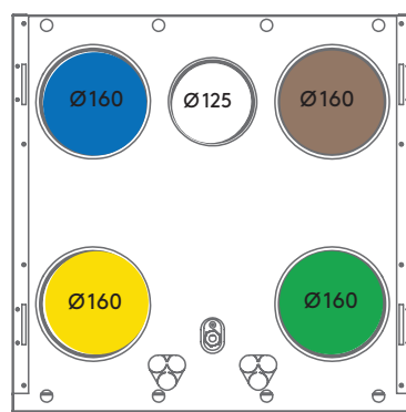
CASA W4 Smart xs R, Rechtsausführung
