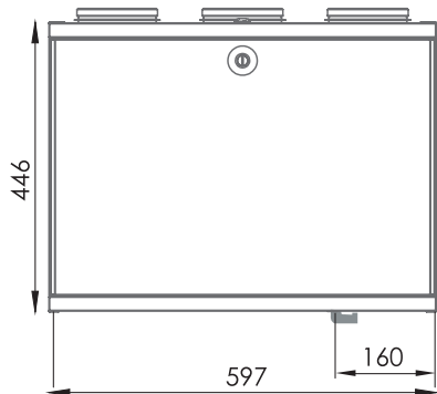
R -modell från framsidan
