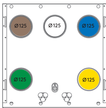
CASA W3 Smart xs L, vänsterutförande
