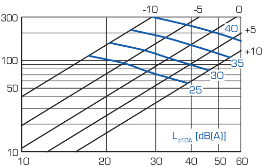
CSB instyckningsdiagram vid forcerad ventilation
