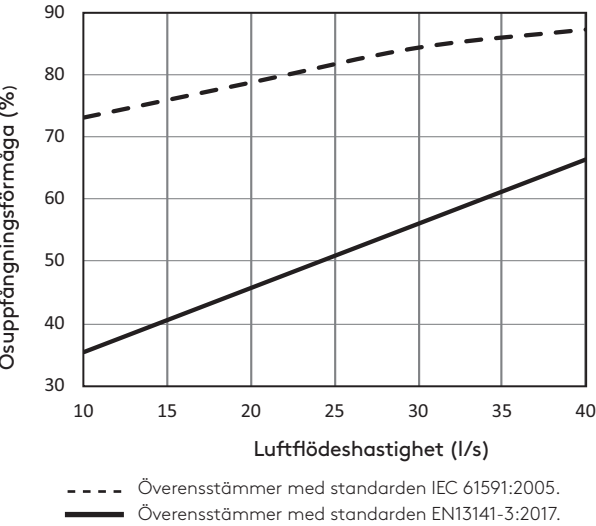
CSB instyckningsdiagram vid forcerad ventilation
