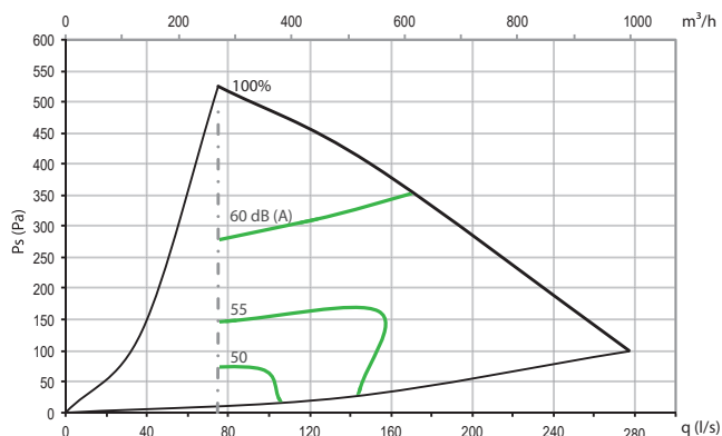
Ljudeffektnivå till utomhusluftskanal
