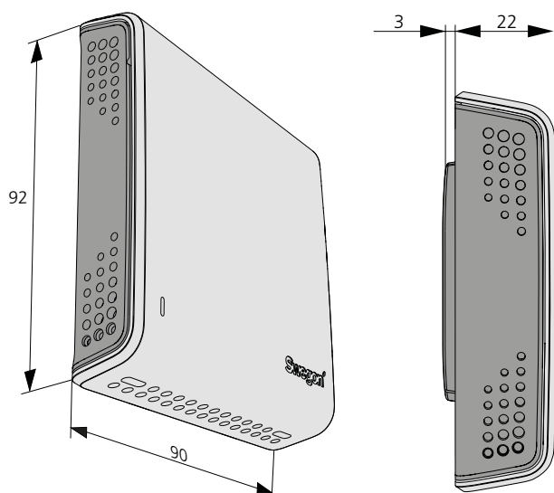
Figur 2. Mått, IAQ.
