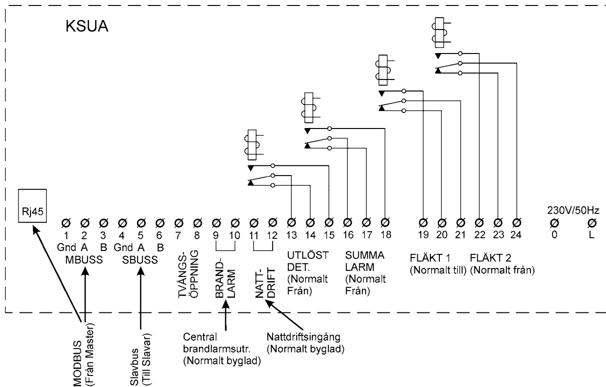
Anslutning av externa enheter.
